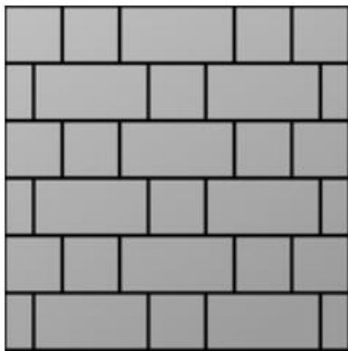
200x100 мм и 100×100 мм "крест"
