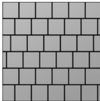
100×100 мм, в разбежку по диагонали
